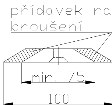
Max. opotřebování/broušení břitů nože
